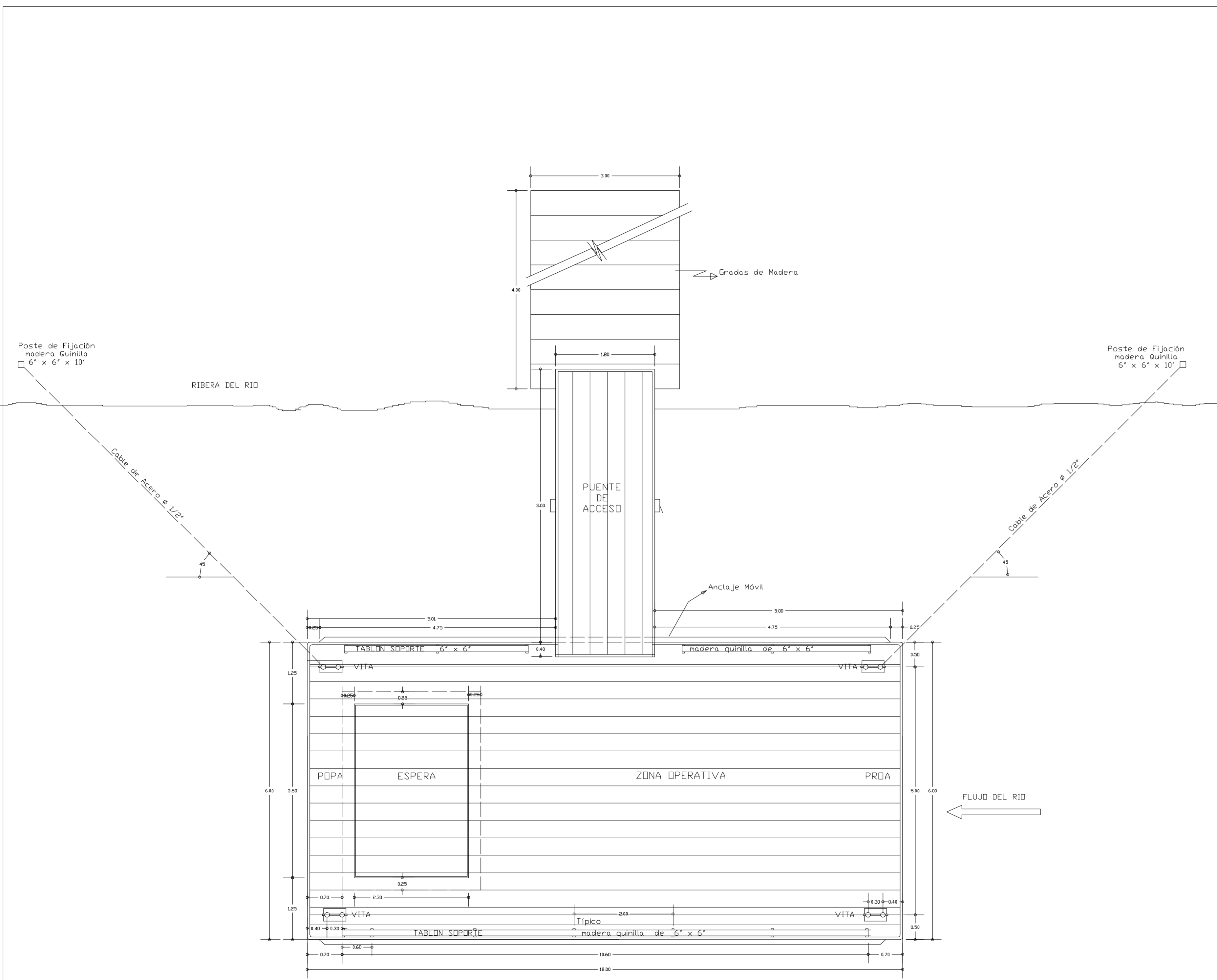
EMBARCADERO FLOTANTE Escala: 1/50
