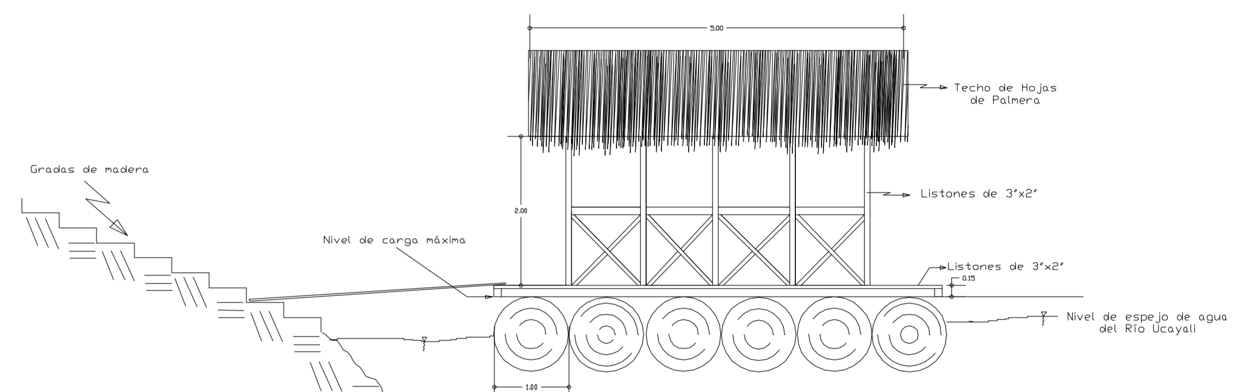
ELEVACION FRONTAL Escala: 1/50
