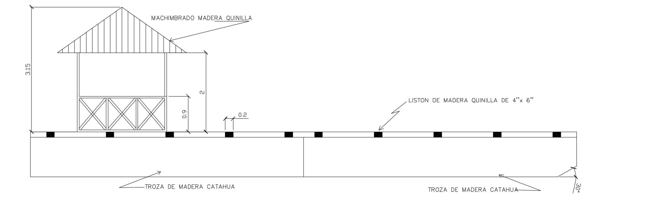
ELEVACION FRONTAL Escala: 1/50
